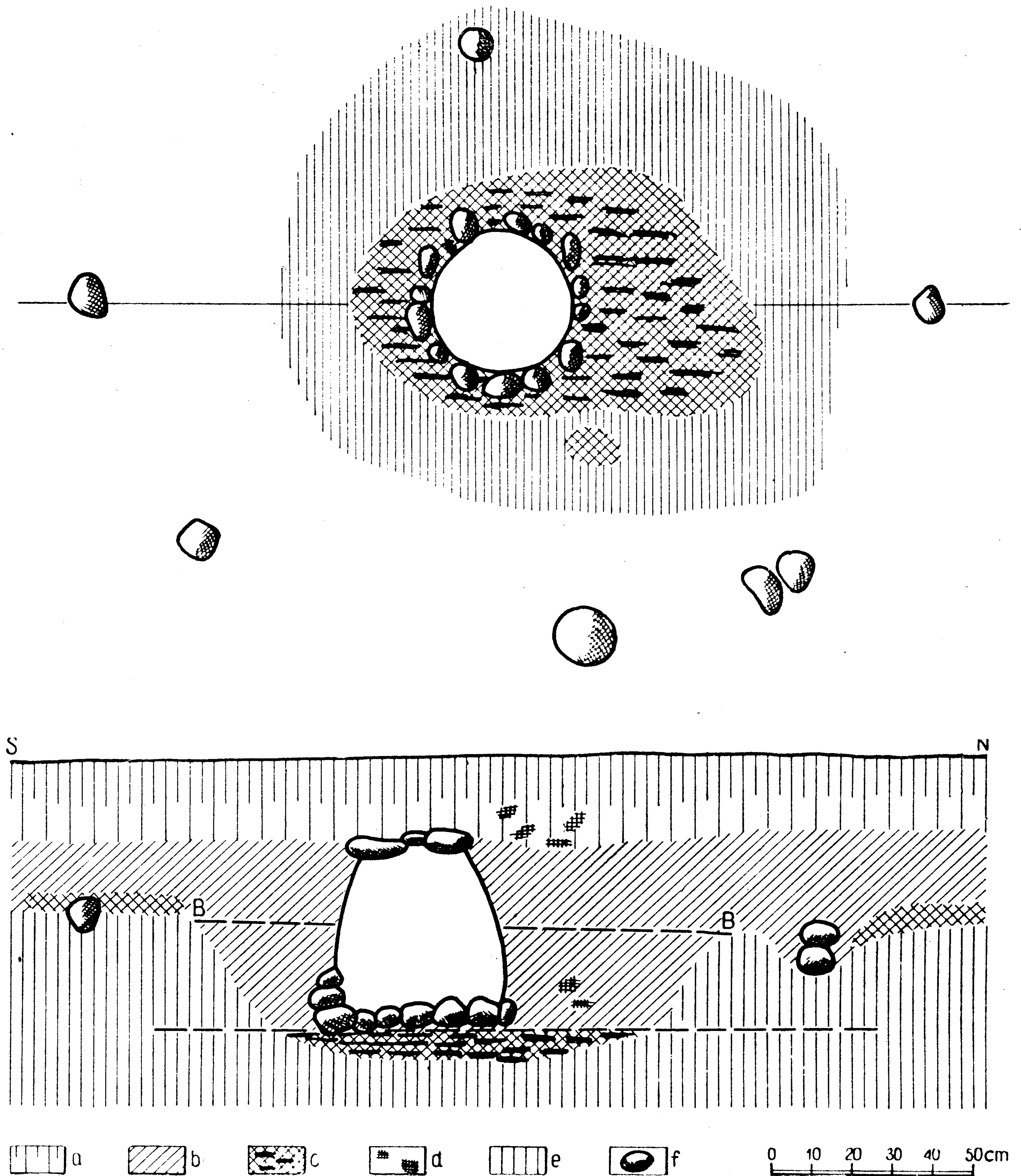
Fig. 2. Transbór, district Mińsk Maz. Plan et profil de la tombe No 49 (Dessiné par M. Curyło) a — humus; b — humus antérieur; c — terre avec des morceaux de charbon de bois; d — fragments de torchis; e — sable claire; f — pierres. B—B— la fosse tombale
